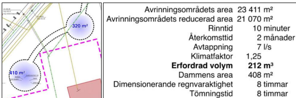
Figur 21 Förutsättningar och beräknad magasinvolym för reningsdammen.
